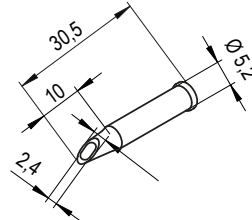
0102YDLF1224/SB geschlitzt, angeschrägt, ID 1,2 mm, AD 2,4 mm
