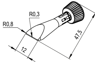
0102SDF06L/SB bleistiftspitz, gebogen, verlängert, 0,6 mm ø
