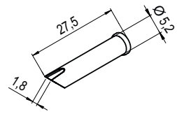
0102YDLF1852 geschlitzt, angeschrägt, ID 1,8 mm, AD 5,2 mm
