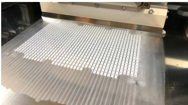
Wärmeleitpaste im Rechteckraster
