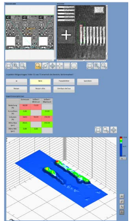
Inspektionsergebnis: Darstellung der Position im Layout, 2D- und 3D-Bild und Ergebnis der Messung mit Soll- und Ist-Werten
