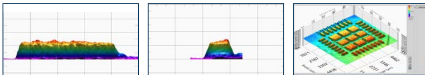
v.l.n.r.: Profilbild des Ergebnisses mit Höhenangabe. Profil- bild – 90 Grad gedreht. Inspektionsergebnis
