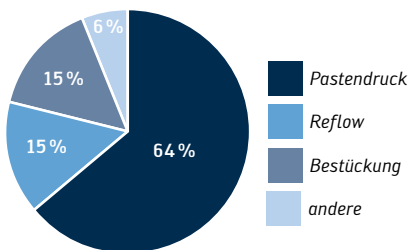
Fehlerverteilung im SMD-Prozess nach C. H. Mangin
